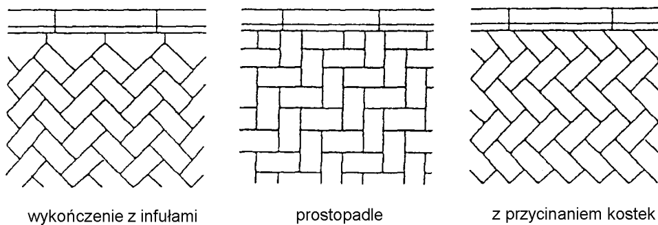
Rys. 4.2. Najczęściej spotykane desenie nawierzchni na wjeździe z betonowej kostki brukowej
