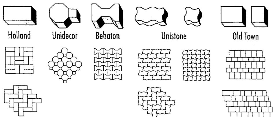
Rys. 4.2. Najczęściej spotykane desenie nawierzchni na wjeździe z betonowej kostki brukowej
